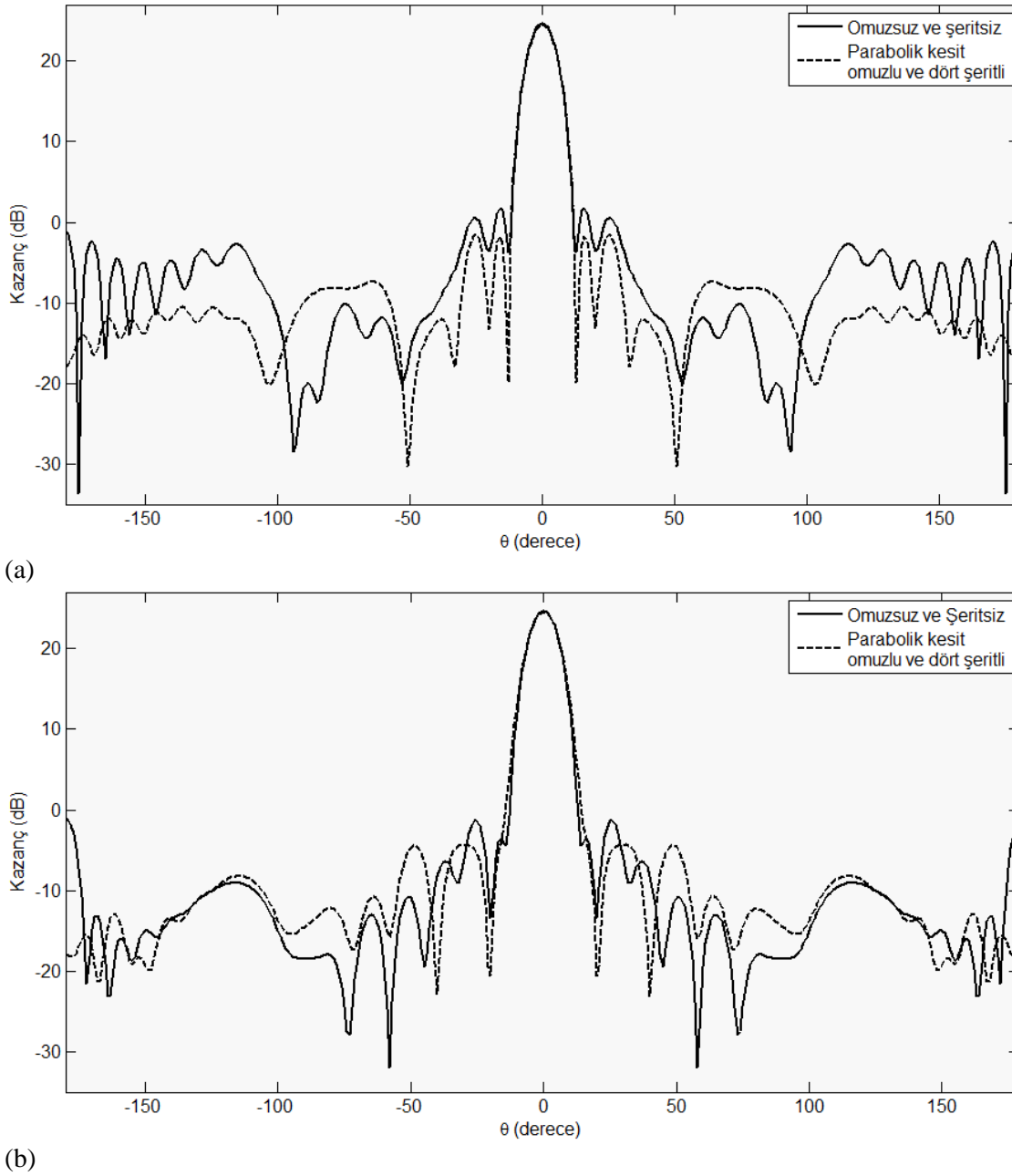
Şekil 6. Işıma desenleri karşılaştırması (a) Yatay düzlem (b) Düşey düzlem
